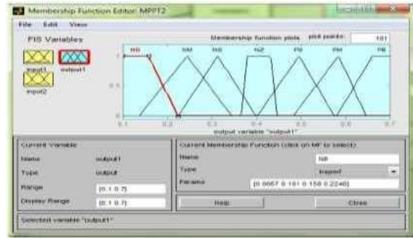
Fig.11 Fuzzy logic output (D)
